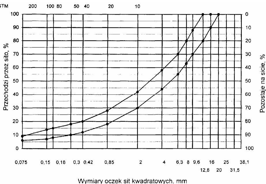
Rys. 3. Krzywe graniczne uziarnienia mieszanki mineralnej BA od 0 do 16 mm do warstwy ścieralnej nawierzchni drogi o obciążeniu ruchem od KR3 do KR6
