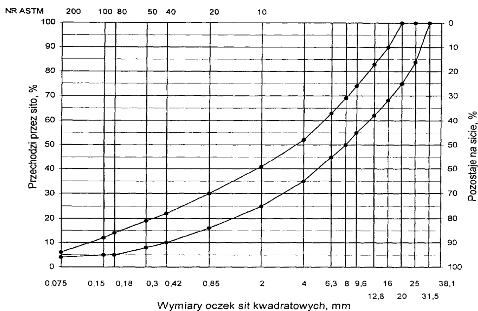
Rys. 5. Krzywe graniczne uziarnienia mieszanek mineralnych BA od 0 do 25 mm do warstwy wiążącej, wyrównawczej i wzmacniającej nawierzchni drogi o obciążeniu ruchem od KR3 do KR6
