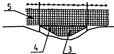
b) zabezpieczenie w postaci kłapy na zawiasie, samoczynnie odchylającej się pod naciskiem przepływających odpadków lub podnoszonej przez pracowników obsługi
