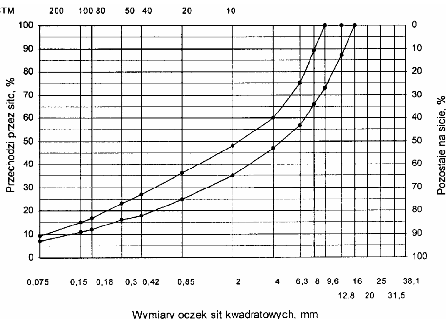
Rys. 4. Krzywe graniczne uziarnienia mieszanki mineralnej BA od 0 do 12,8 mm do warstwy ścieralnej nawierzchni drogi o obciążeniu ruchem od KR3 do KR6
