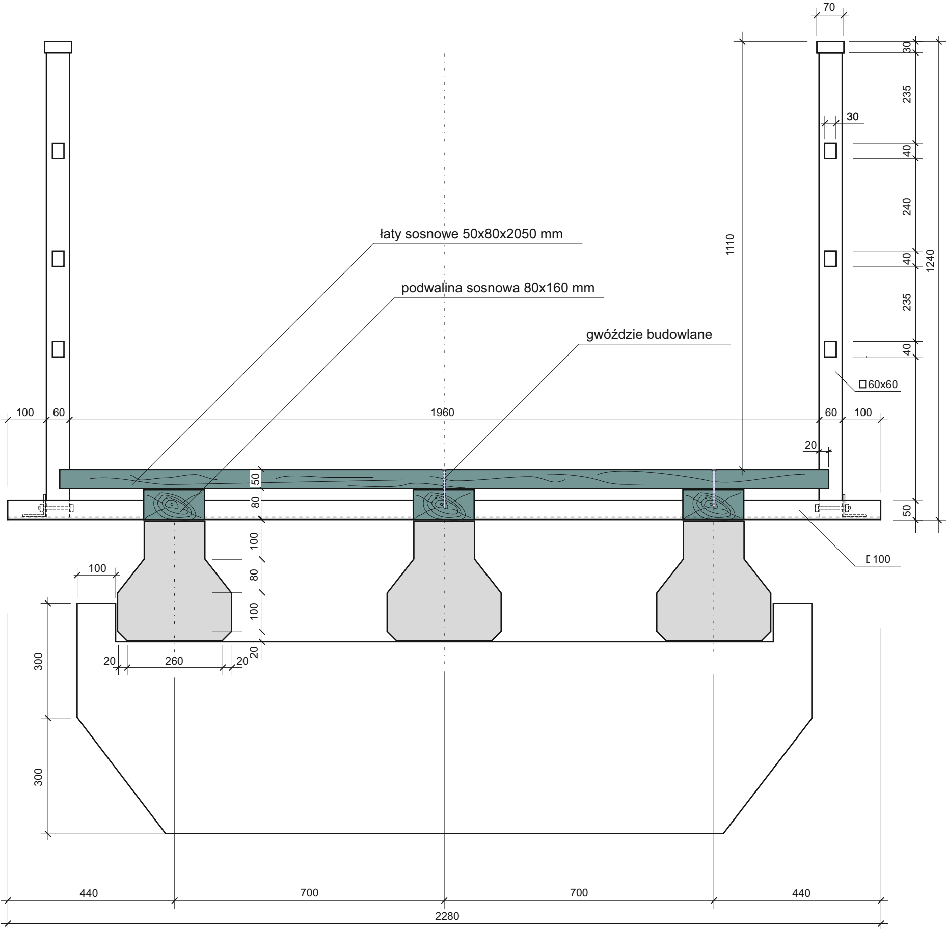
PRZEKRÓJ A-A
